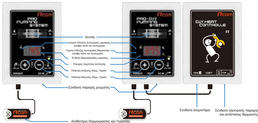
τρόπος συνδέσης των συσκευών αυτόματης ύγρανσης και θερμοκρασίας σε εκκολαπτική μηχανή
